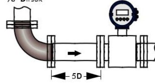
90° Dirsek
