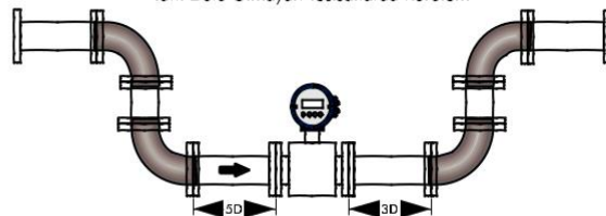
Tam Dolu Olmayan Tesisatlarda Kurulum
